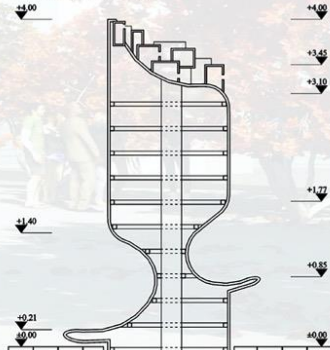
AA Kesiti
